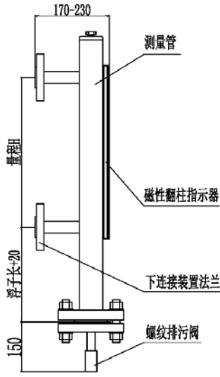
UHC 侧装磁性浮子式液位计 (普通型、高温型、高压型)
