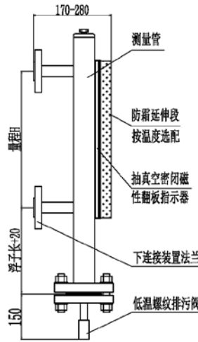
UHC 侧装磁性浮子式液位计 (低温型)
