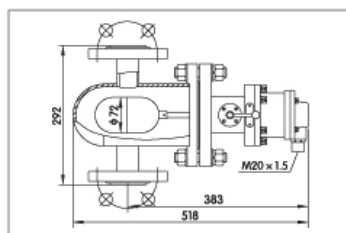
UQKS-104 型外型及结构尺寸图
