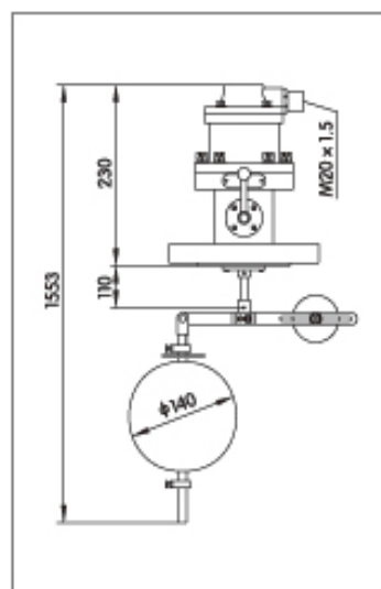
UQKS-103 型外型及结构尺寸图
