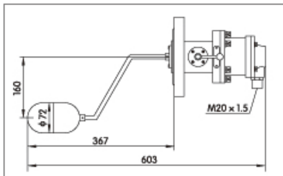
UQKS-1011 型外型及结构尺寸图
