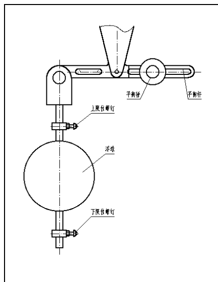
UQKS-103 型 浮球液位控制器控制范围调整图
