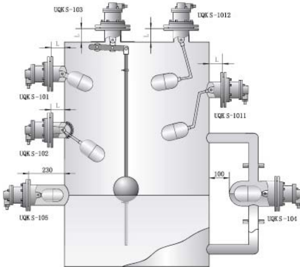
UQKS-100 系列浮球液位控制器安装示意图
