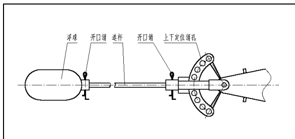
UQKS-102 型浮球液位控制器测量范围调整图
