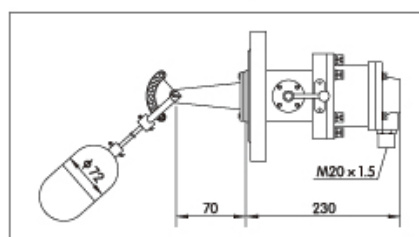
UQKS-1012 型外型及结构尺寸图
