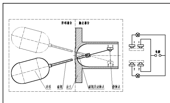
UQK—100 型系列浮球液位控制器结构原理图
