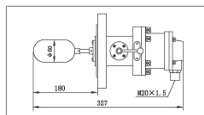
UQKS-103 型外型及结构尺寸图
