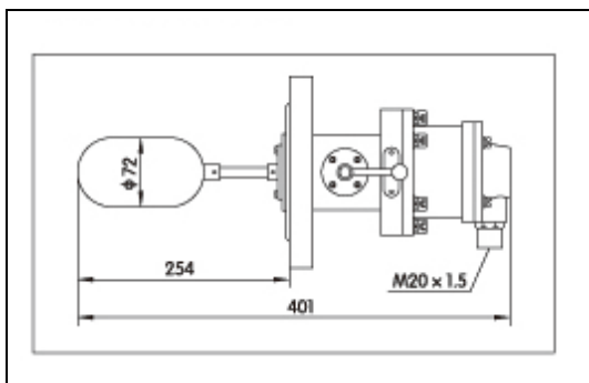
UQKS-101 型外型及结构尺寸图
