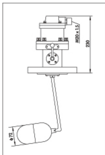
UQKS-1012 型外型及结构尺寸图
